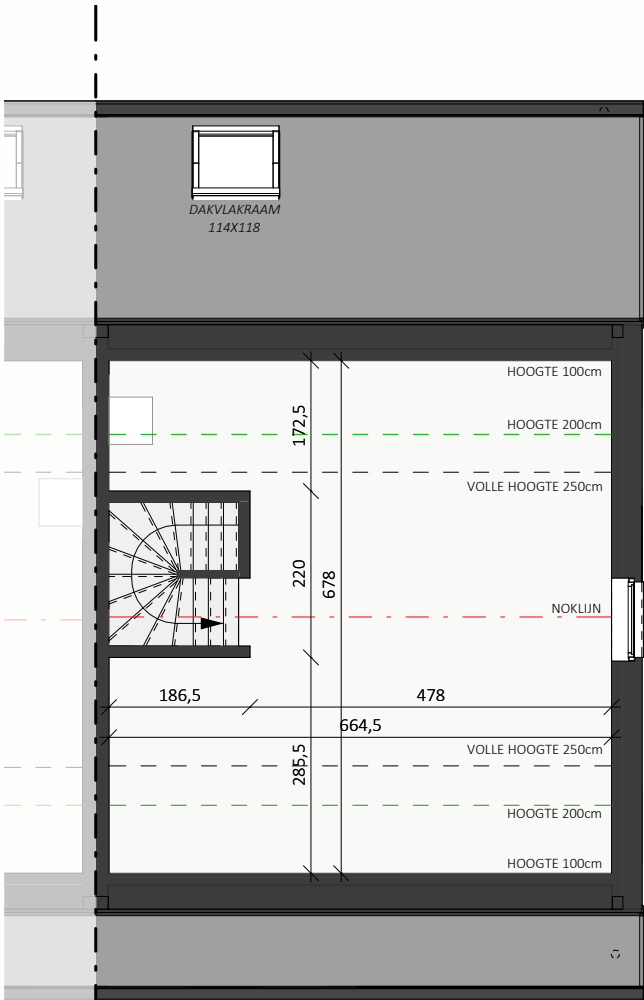
2e VERDIEPING
