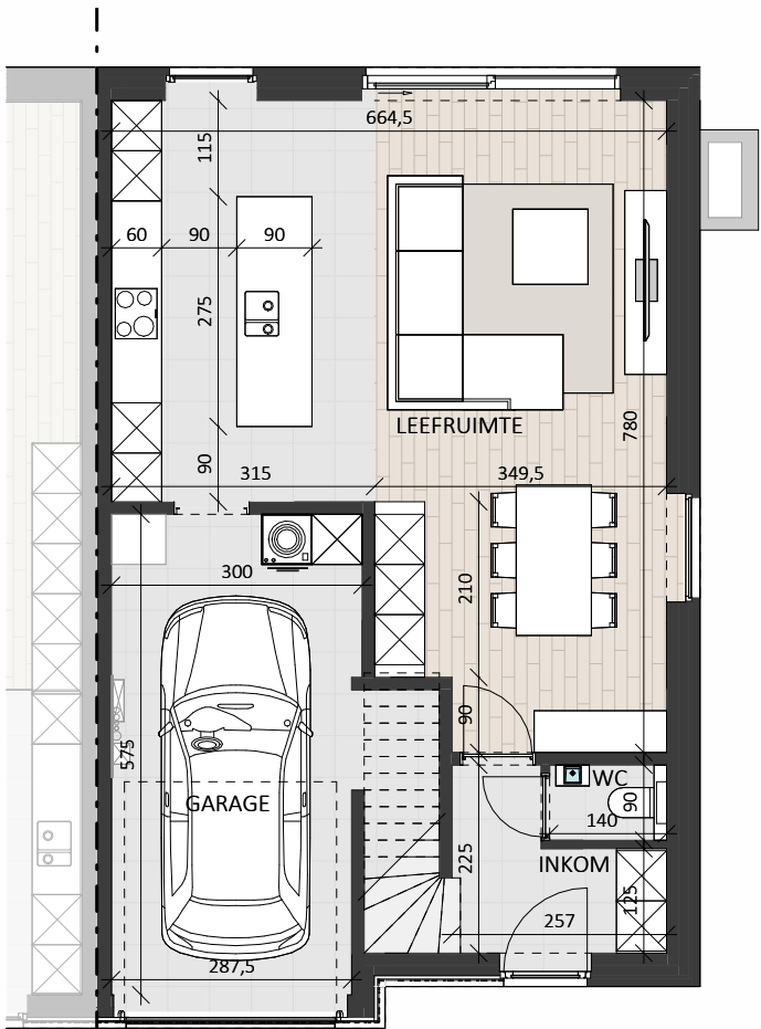
GELIJKVLOERS
